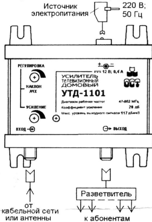
Рисунок 1 - Общий вид и подключение усилителя к внешним устройствам
