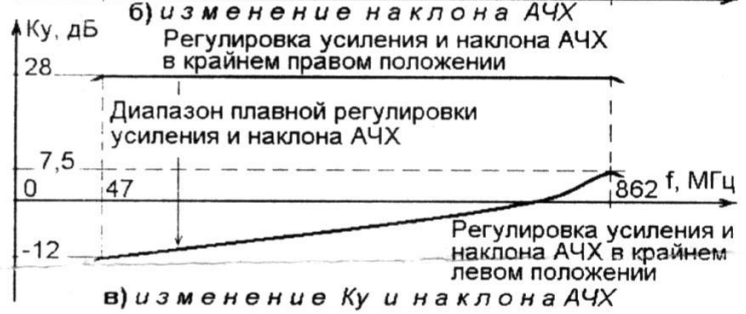
Рисунок 2 - Изменение амплитудно-частотной характеристики (АЧХ) усилителя с помощью органов плавной регулировки
